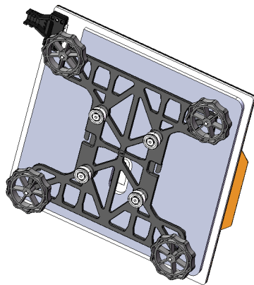
20.204.0123 底部滑块板套件 Base Slide Block Kit
